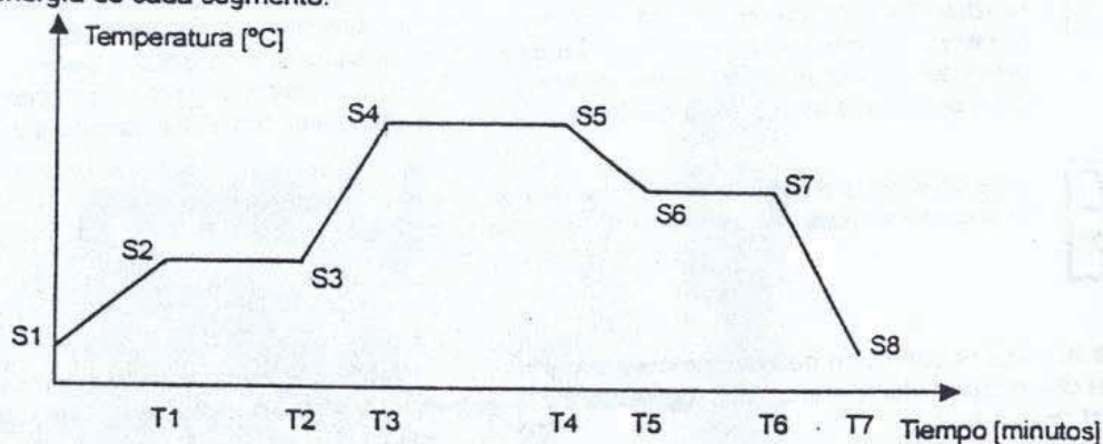
Diagrama de set point en función del tiempo para un ciclo de rampas y mesetas.
